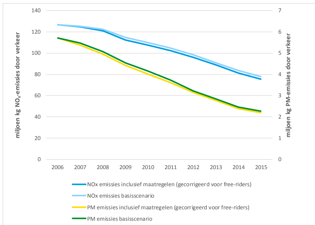
Figuur 3 - Verloop van wegverkeersemissies over de tijd met en zonder maatregelen (mln kg)
