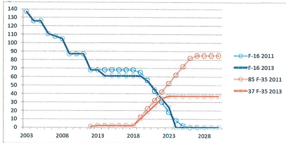
Figuur 3 Invoerreeks F-35 en afvoerreeks F-16. Bron: Jaarrapportage Vervanging F-16 2013
